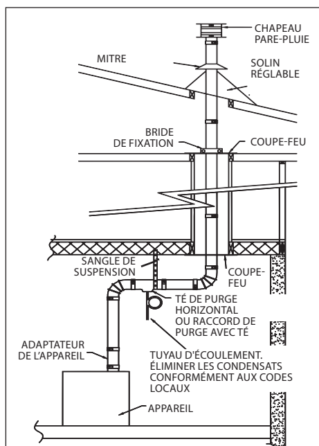
Installation verticale traversant un toit
