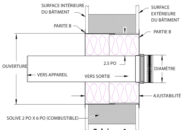
Schéma 4 - Installation de la virole murale simple
