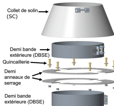
Schéma 66a - Détail de la section des haubans
