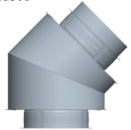
Schéma 35d: Coude 45°
