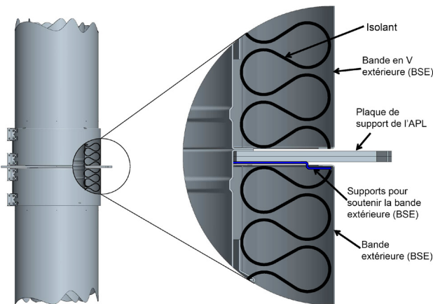
Schéma 46 - Étape 3 de l'installation de l'APL
