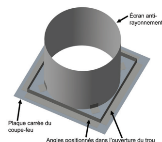
Schéma 58a - Coupe-feu de toit (RT)
