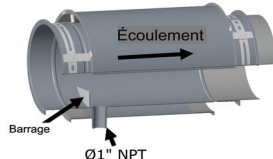
Schéma 73 - Longueur de drainage horizontale (HDL)
