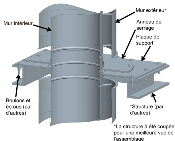
Schéma 41a - Plaque d'ancrage sur la charpente
