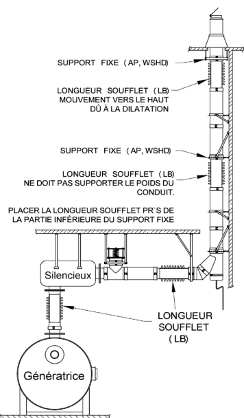
Schéma 53- Localisation des longueurs soufflet
