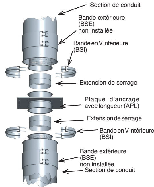
Schéma 44 - Étape 1 de l'installation de l'APL
