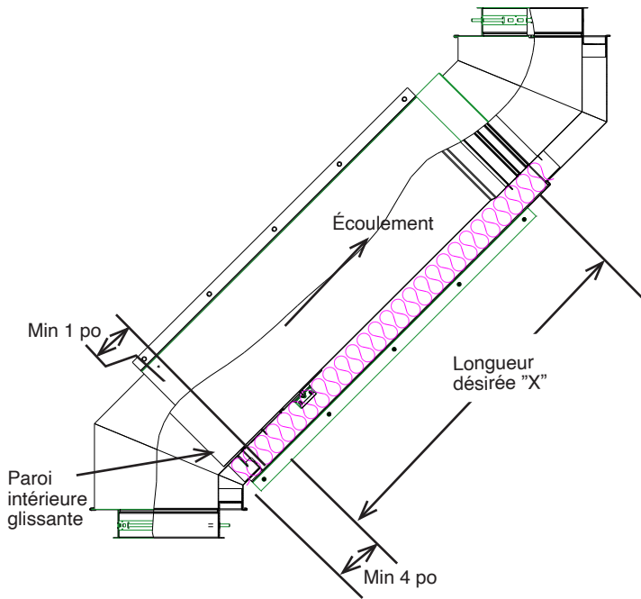
Schéma 22 - Détails de chevauchement de la longueur variable
