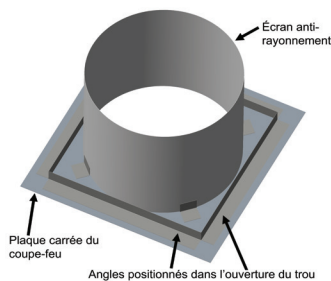
Schéma 112: Coupe-feu de toit (RT)
