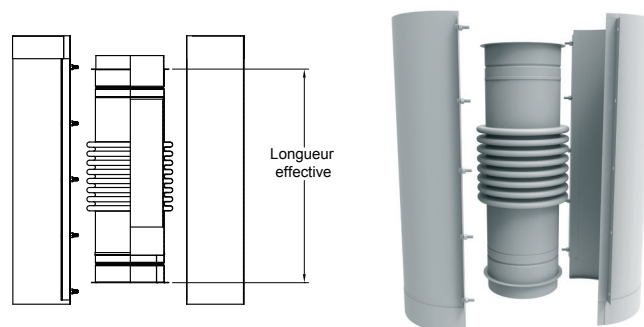
Schéma 12 - Longueur soufflet
