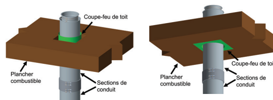
Schéma 58b - Coupe-feu installé
