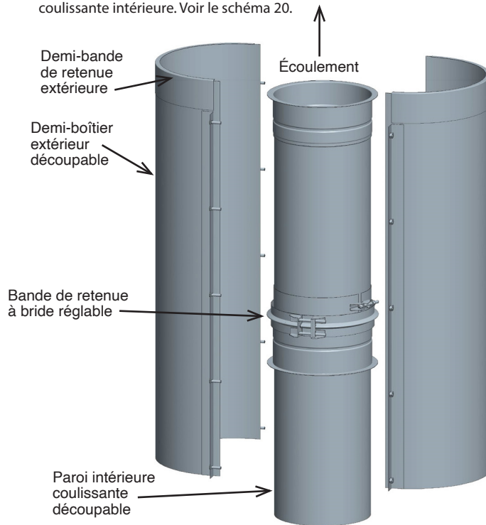
Schéma 20 - Longueur variable
