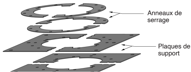
Schéma 40 - Plaque d'ancrage
