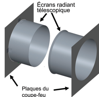
Schéma 114: Coupe-feu mural (WT)
