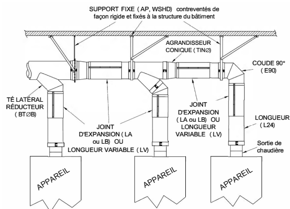
Schéma 54- Support pour plusieurs tés
