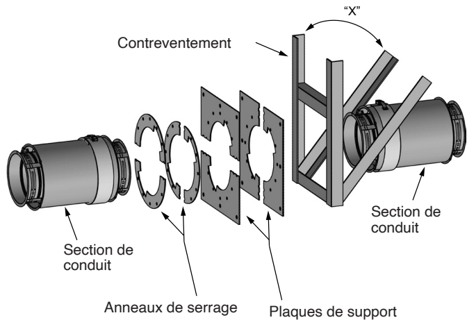
Schéma 42 - Plaque d'ancrage sur contreventement
