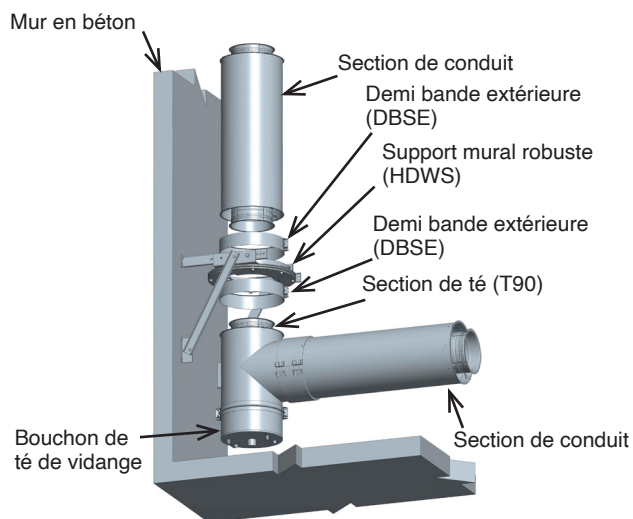
Schéma 55- Support de té en suspension
