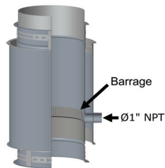
Schéma 72 - Longueur de drainage (DL)
