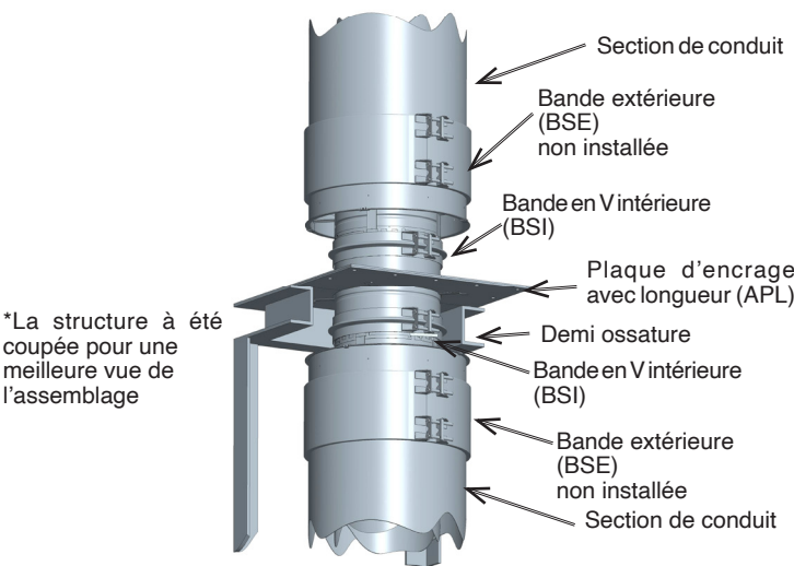
Schéma 45 - Étape 2 de l'installation de l'APL
