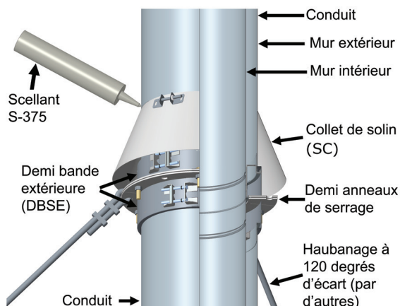
Schéma 66b - Haubannage installé
