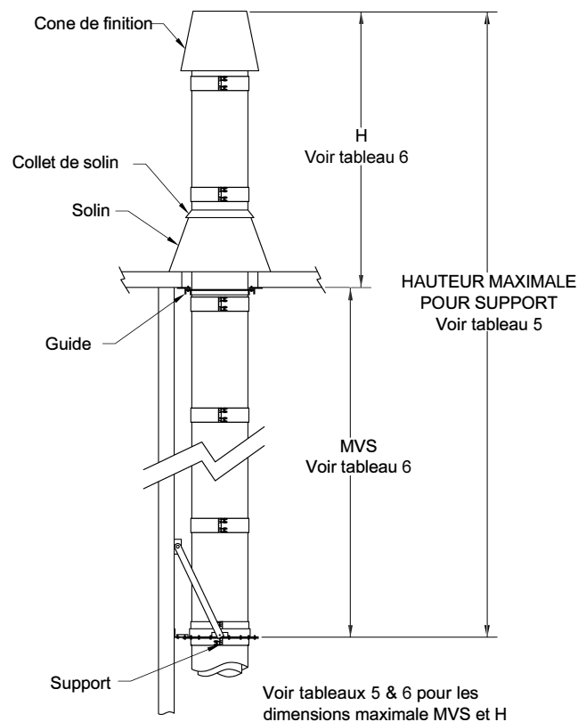
Schéma 4 - Hauteur autoportante maximale
