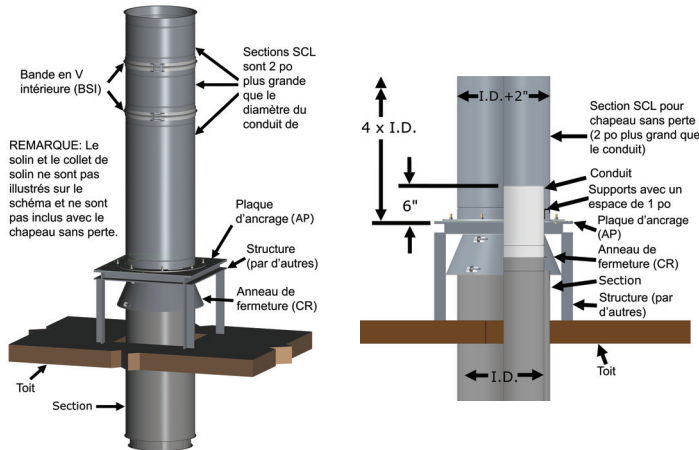
Schéma 71b & c - Capuchon sans perte (NLC) installé pour I.D. de 14" à 36"
