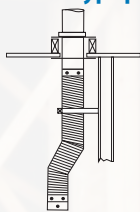
DÉVIATION TRAVERSANT UN PLAFOND
